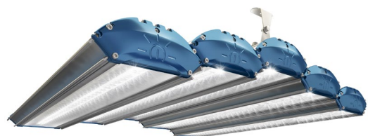
Габариты, ДхШхВ, мм: 745х727х185 Масса, кг: 14,44
