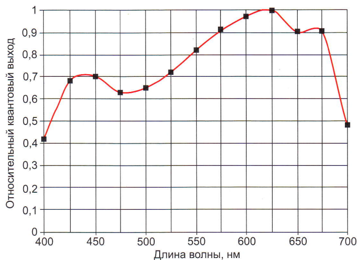
Рис. 2. Влияние спектра на фотосинтез для культурных растений
