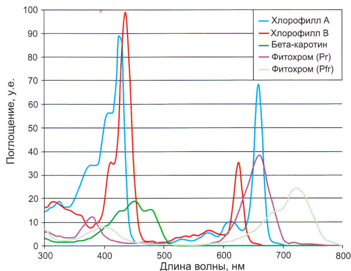
Рис. 1. Спектральные характеристики поглощения фотопигментов
