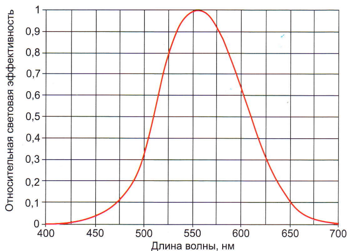
Рис. 4. CIE 1931 относительная световая эффективность V(l)
